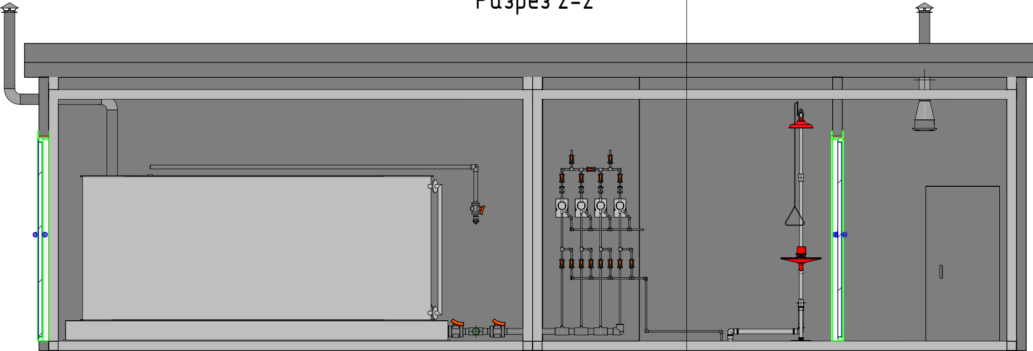
Разрез 2-2
